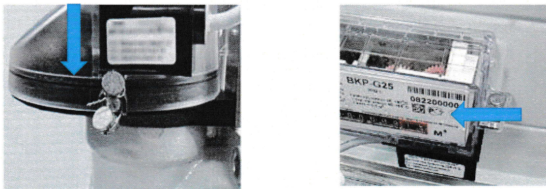
Рисунок 5 – Схема пломбировки от несанкционированного доступа места присоединения датчика импульсов, обозначение места нанесения знака поверки счетчика газа
