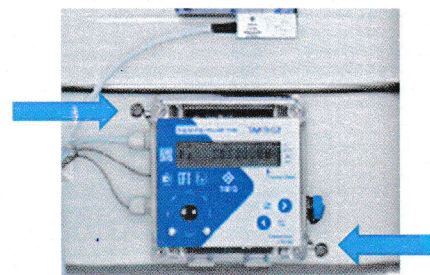
Монтаж термопреобразователя сопротивления Pt500 (500П) в потоке газа
