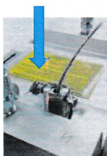
Монтаж термопреобразователя сопротивления Pt500 (500П) в потоке газа
