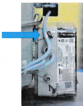
Монтаж термопреобразователя сопротивления Pt500 (500П) на корпусе счетчика
